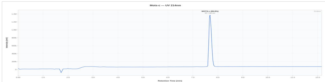
Mots-c 10mg - 0326-A: UV Chromatogram
